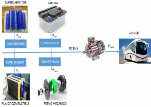
Fig. 1. Esquema del sistema de propulsión del vehículo
