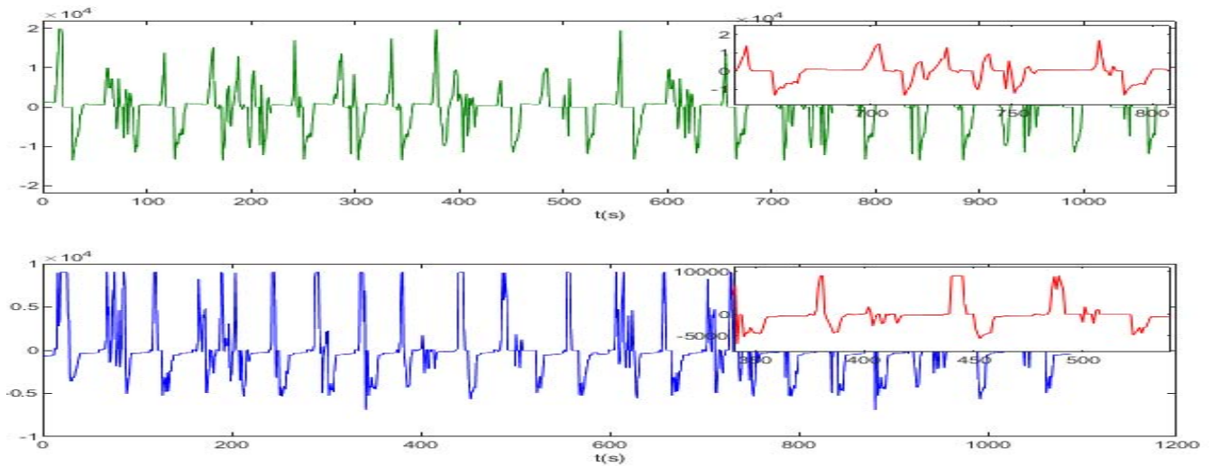
Fig. 16. Potencia de los componentes del sistema de almacenamiento con el controlador REMPC para cumplir el BADC.
