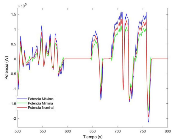
Fig. 7. Sección de potencia máxima, mínima y real requerida para cumplir el BADC
