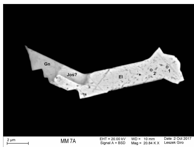
Fig. 11. Pegmatyt z kamieniołomu Kamienna Góra. Powiększony fragment fig. 10. Kryształ elektrumu (El) z galeną (Gn) i prawdopodobnie jositite? (Jos) (obraz BSE)
