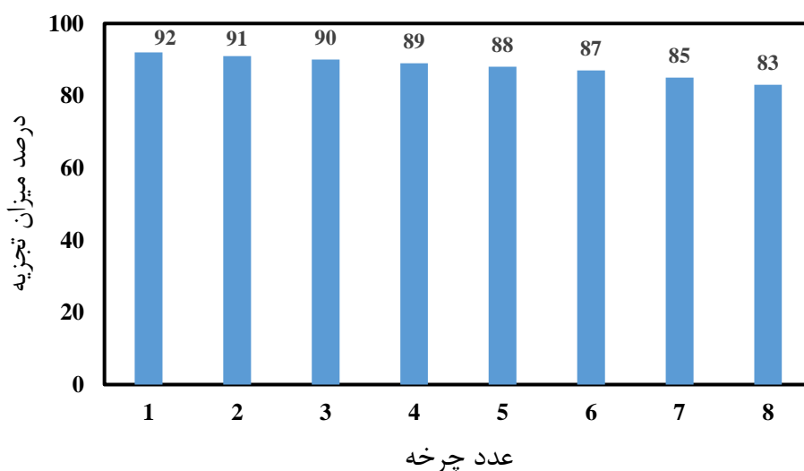
شکل ۱۰: تأثیر استفاده مجدد کاتالیست بر تجزیه متریئیدازول
