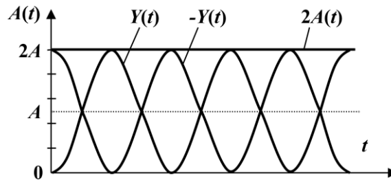
Рис. 3. Отримання амплітуди 2A(t) сигналу S(t) в двоканальному піковому АД (форма обвідної – прямокутна)
