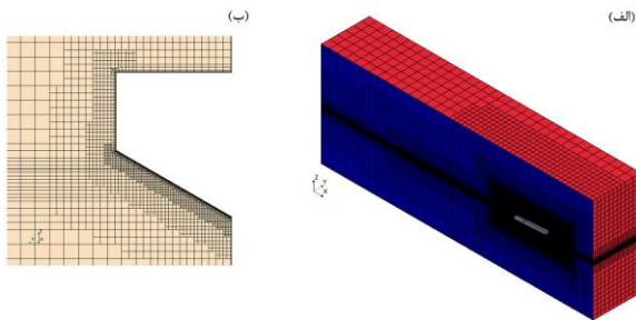
شکل ۳: (الف) نمای سه بعدی از محدوده محاسباتی شبکه بندی شده (ب) نمای دوبعدی در صفحه yz در اطراف بدنه شناور
