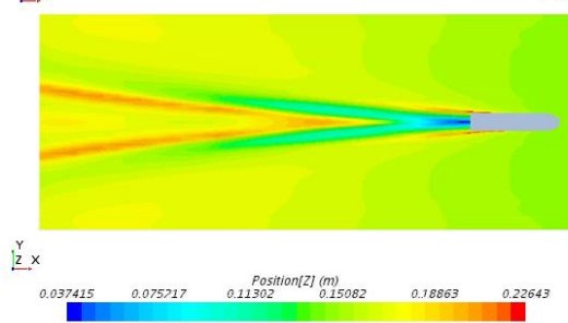
شکل ۸: الگوی موج تولید شده اطراف بدنه شناور در سرعت های مختلف
