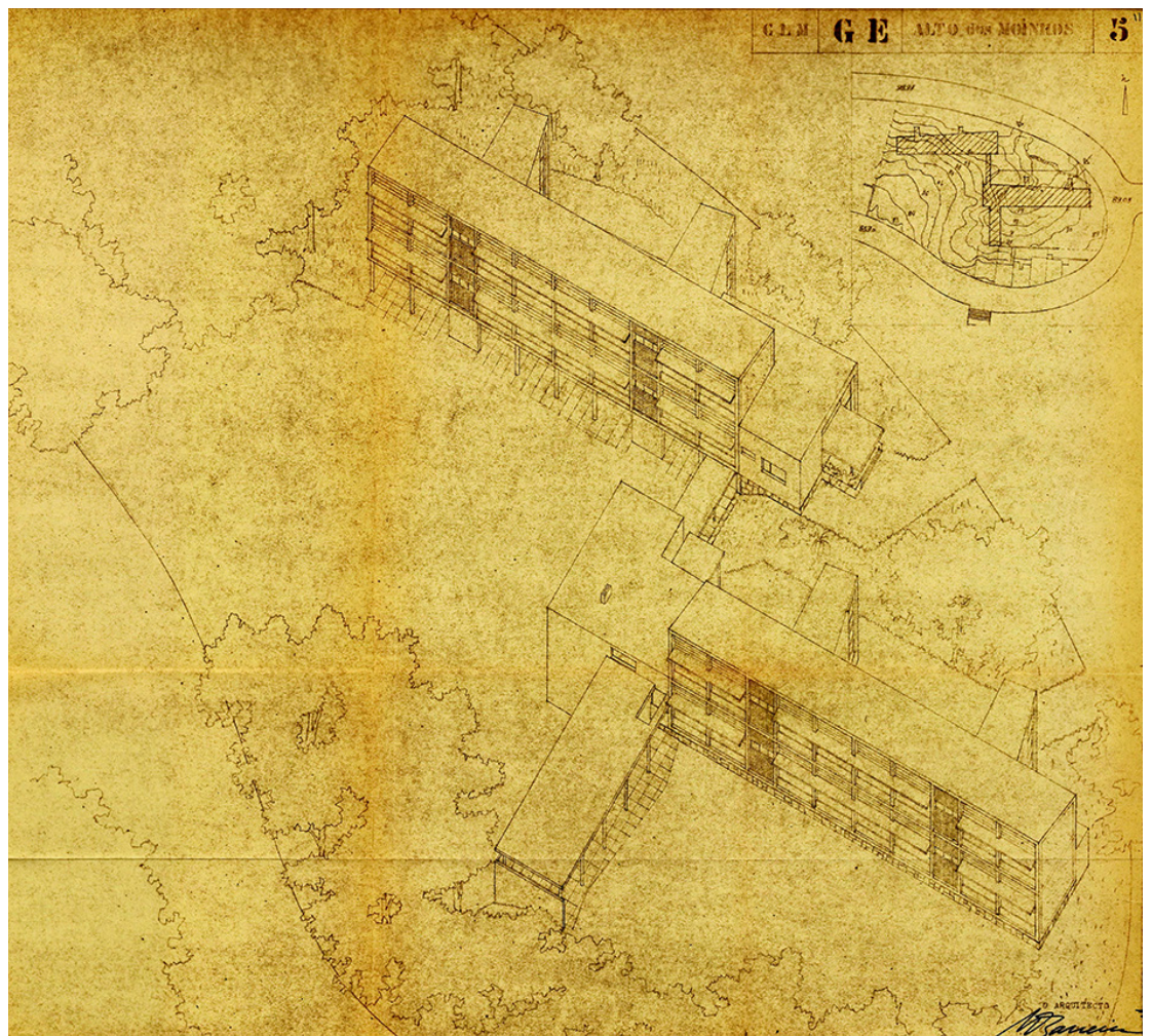
Figura 10 Planta de localização do Grupo Escolar para o Alto dos Moinhos, arquiteto Cândido Palma de Melo, [1953]. Arquivo Municipal de Lisboa, PT/AMLSB/CMLSBAH/PURB/002/04064, página 11.
