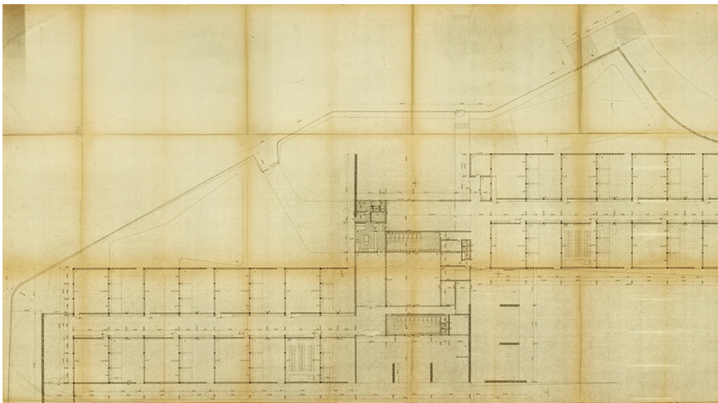
Figura 15 Metade da planta do piso único do Grupo Escolar da Célula 8 de Alvalade, arquiteto Ruy Jervis Athouguia, [1957]. Arquivo Municipal de Lisboa, PT/AMLSB/CMLSB/BAH/PURB/002/04080, página 3.
