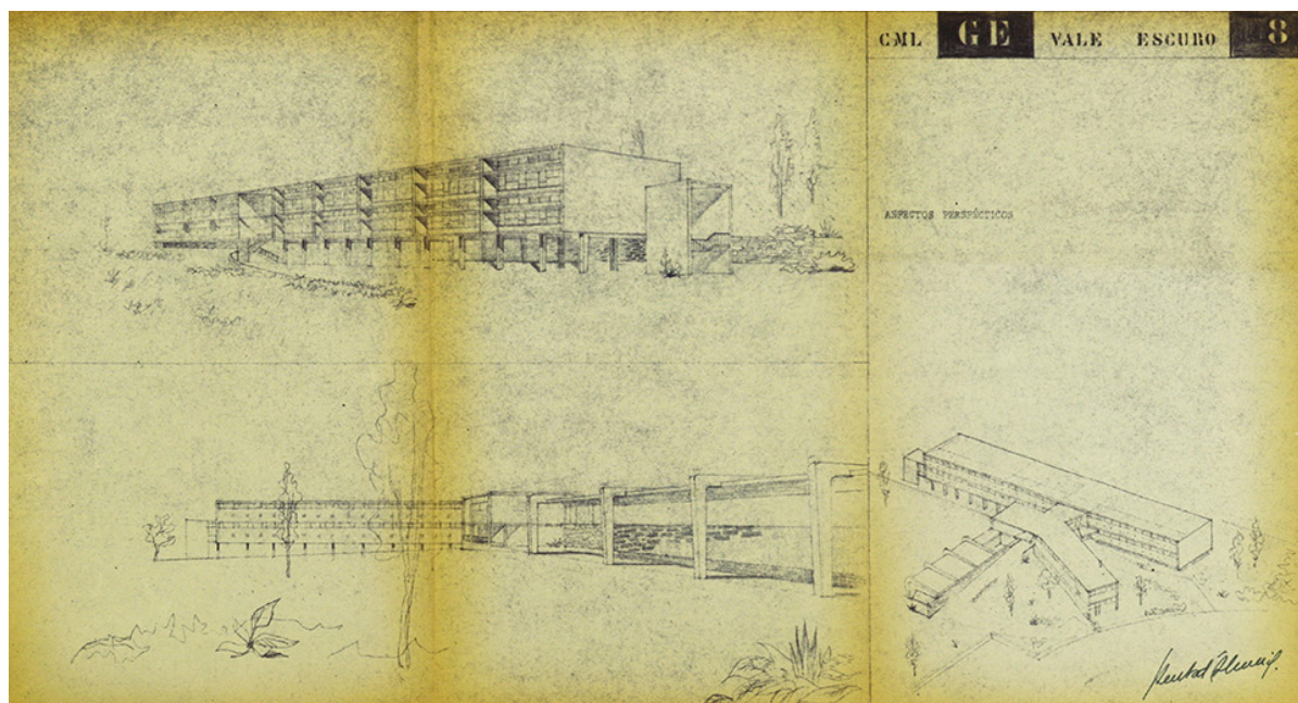
Figura 18 "Aspectos Perspéticos" do Grupo Escolar de Vale Escuro, arquiteto Bento d'Almeida, 1953-08-05. Arquivo municipal de Lisboa, PT/AMLSB/CMLSAH/PURB/002/04071, página 14.
